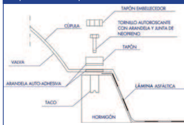
Esquema de montaje sobre base-obra.
